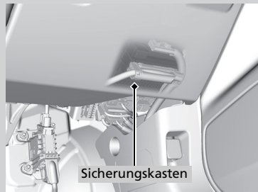
Rechtslenker-Ausführung
